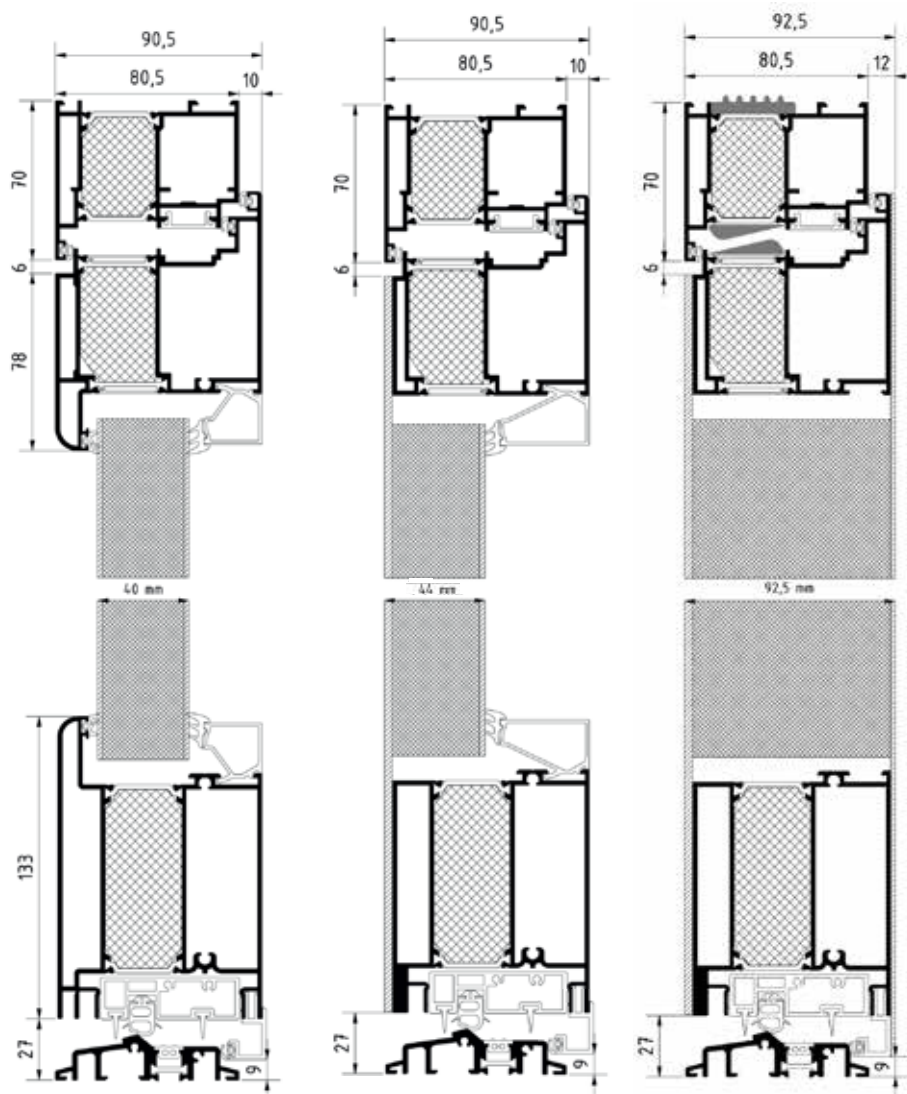
480 SELECTION Standard mit gerundetem Türflügel Abb. mit Einsatzfüllung
